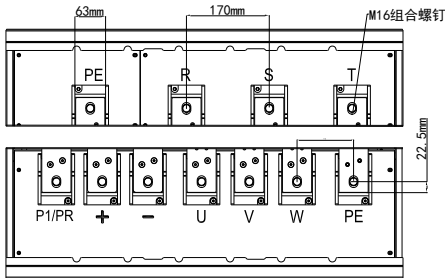
图 3-13 三相 355-450kW 主回路端子分布及尺寸图
