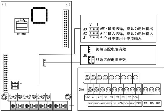
图 3-16 控制回路端子布置图
