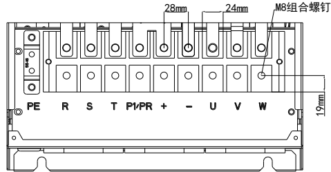
图 3-8 三相 45-55kW 主回路端子分布及尺寸图
