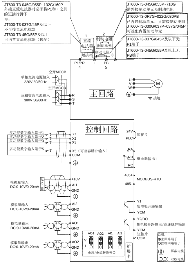
图 3-2 驱动器典型接线示意图
