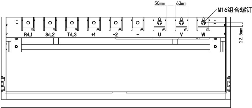
图 3-15 三相 630-710kW 主回路端子分布及尺寸图
