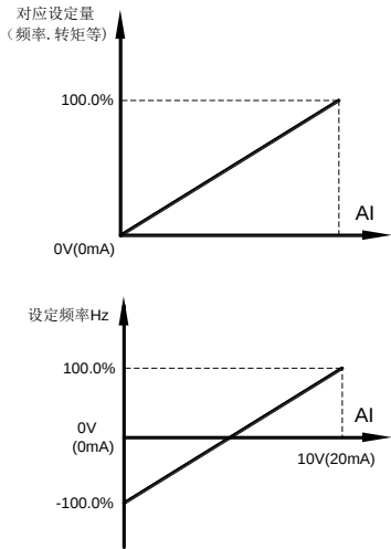
图 6-16 模拟量偏置示意图
