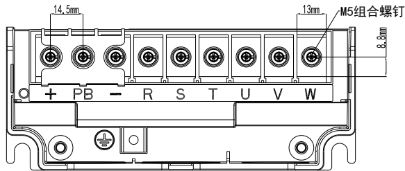
图 3-5 三相 7.5-11kW 主回路端子分布及尺寸图
