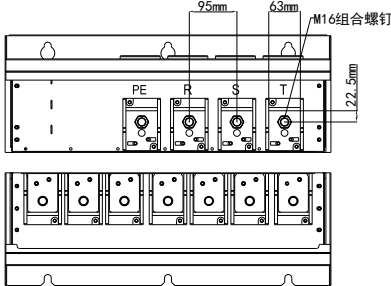
图 3-12 三相 250-315kW 主回路端子分布及尺寸图
