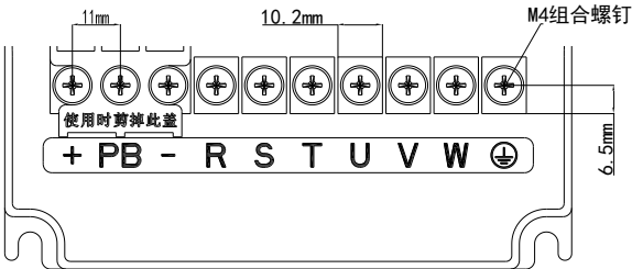
图 3-4 三相 4.0-5.5kW 主回路端子分布及尺寸图
