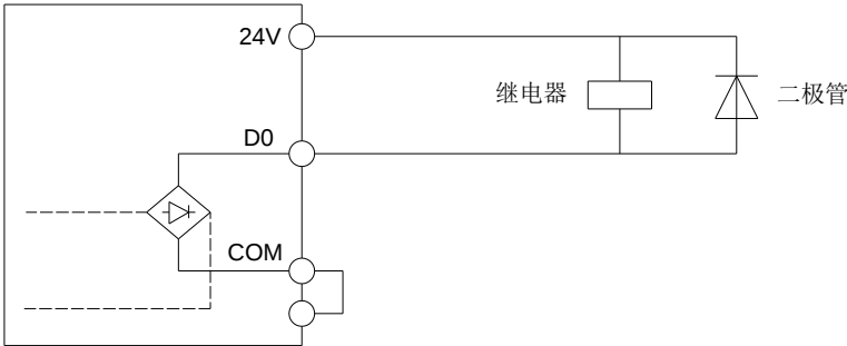
图 3-21 数字输出端子接线示意图
