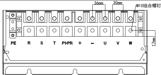
图 3-9 三相 75-90kW 主回路端子分布及尺寸图
