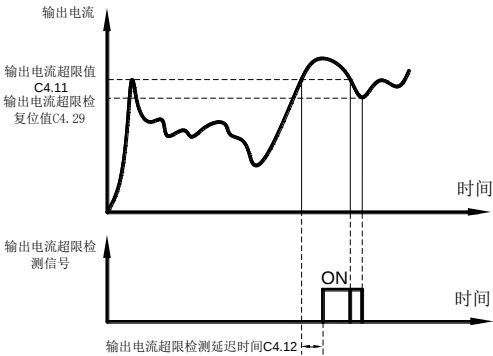
图 6-21 输出电流超限示意图
