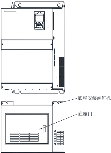
图 1-7 柜式安装示意图
