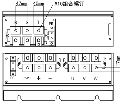
图 3-10 三相 110-160kW 主回路端子分布及尺寸图
