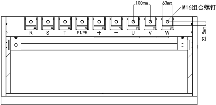
图 3-14 三相 500-560kW 主回路端子分布及尺寸图
