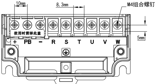
图 3-3 三相 0.75-2.2kW 主回路端子分布及尺寸图
