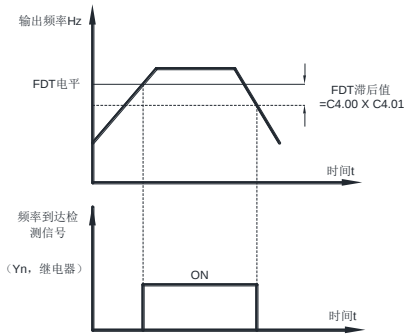
图 6-18 频率 FDT 示意图
