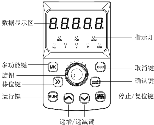
图 4-1 键盘示意图
