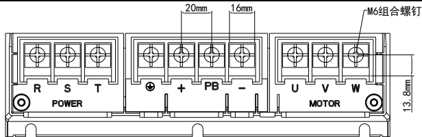
图 3-7 三相 30-37kW 主回路端子分布及尺寸图
