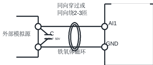
图 3-18 模拟量输入端子处理接线图
