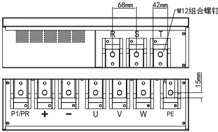
图 3-11 三相 200-220kW 主回路端子分布及尺寸图
