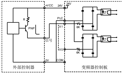
图 3-22 源型接线方式
