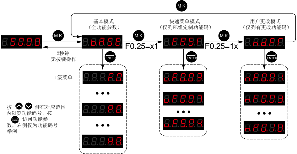
图 4-5 菜单切换
