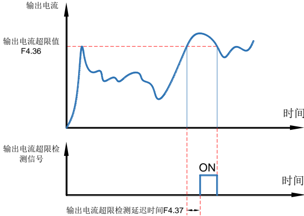
图 7-15 输出电流超限示意图
