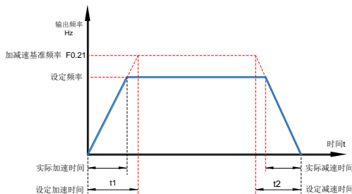
图 7-2 加减速时间示意图
