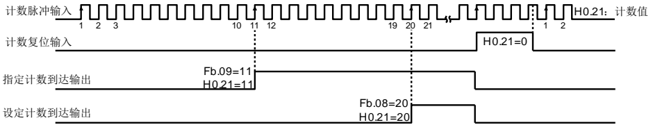
图 7-27 计数功能示意图
