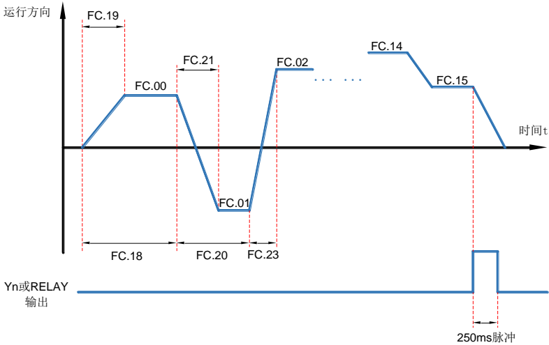
图 7-28 PLC 运行示意图
