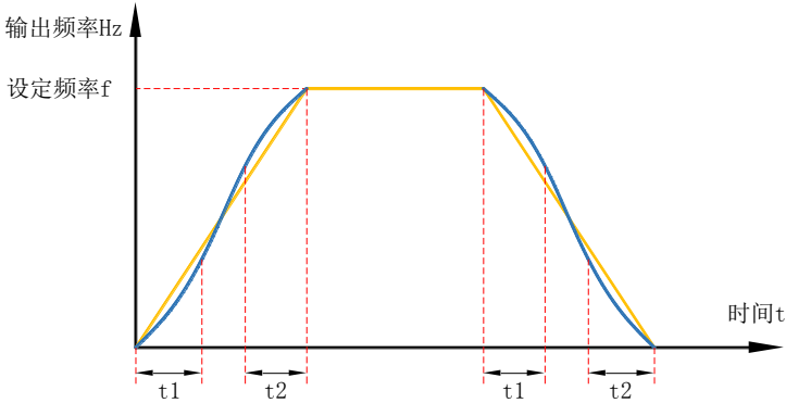
图 7-20 S 加减速曲线 A 示意图
