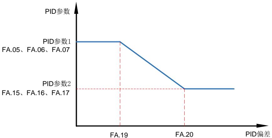
图 7-24 PID 切换示意图
