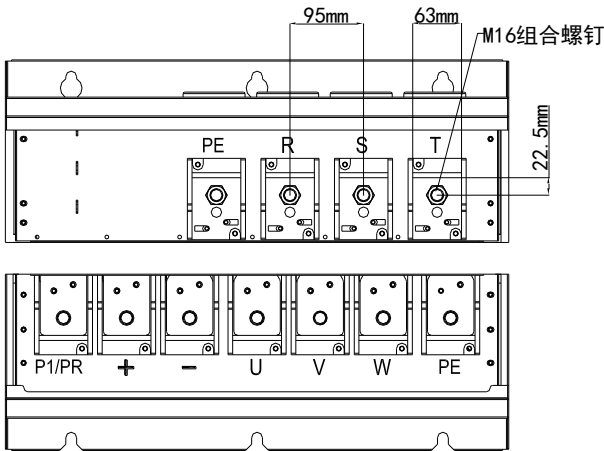
图 3-14 三相 250-315kW 主回路端子分布及尺寸图
