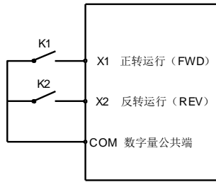
图 7-3 两线运行模式 1
