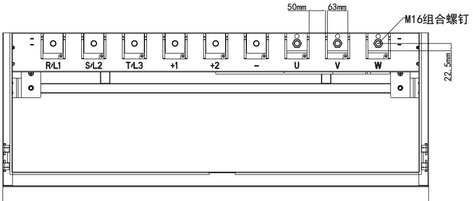
图 3-17 三相 630-710kW 主回路端子分布及尺寸图
