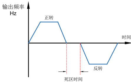
图 7-9 正反转死区时间示意图
