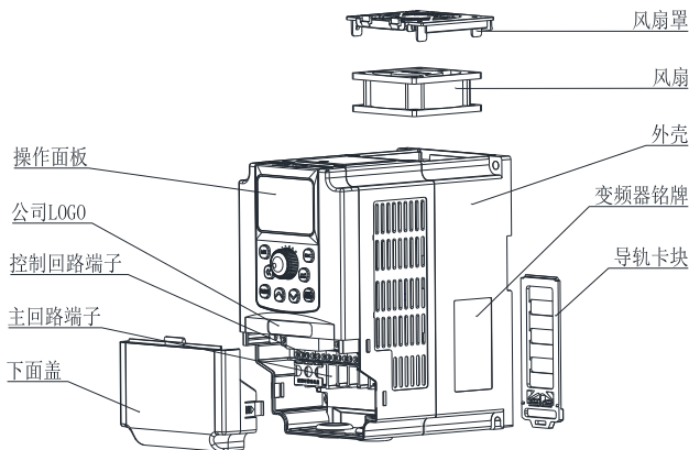
图 1-3 塑胶外壳机型各部分名称
