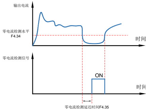
图 7-14 零电流检测示意图
