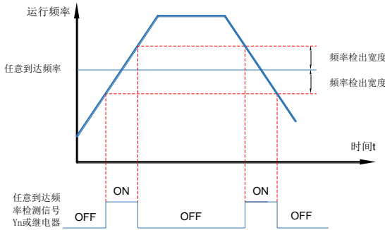
图 7-13 任意频率到达示意图
