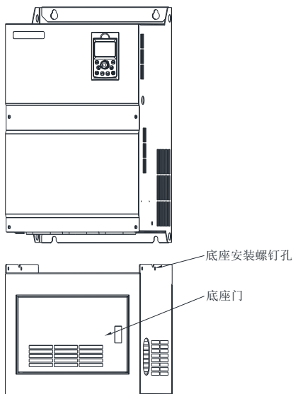
图 1-7 柜式安装示意图
