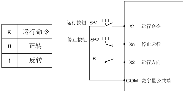
图 7-6 三线运行模式 2
