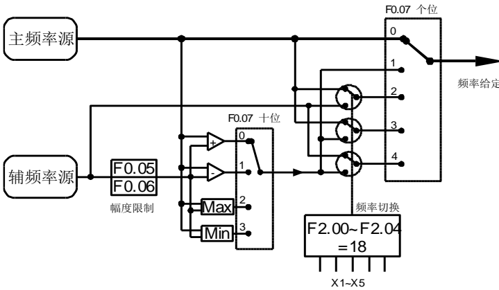
图 7-1 频率给定方式示意图
