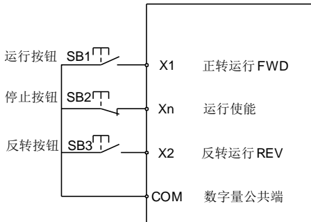
图 7-5 三线运行模式 1
