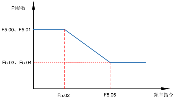
图 7-17 矢量控制 PI 切换
