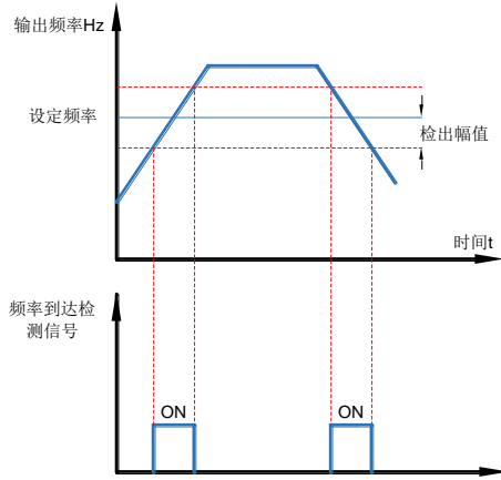
图 7-11 频率到达示意图
