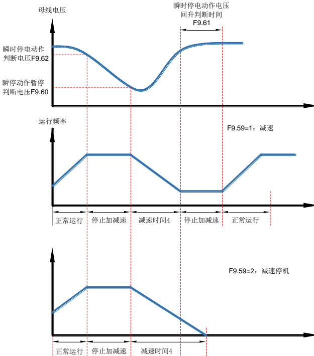
图 7-23 瞬时停电动作示意图
