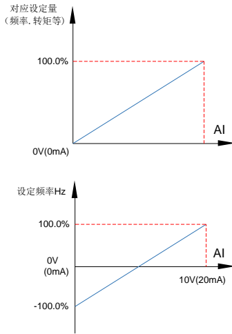
图 7-7 模拟量偏置示意图
