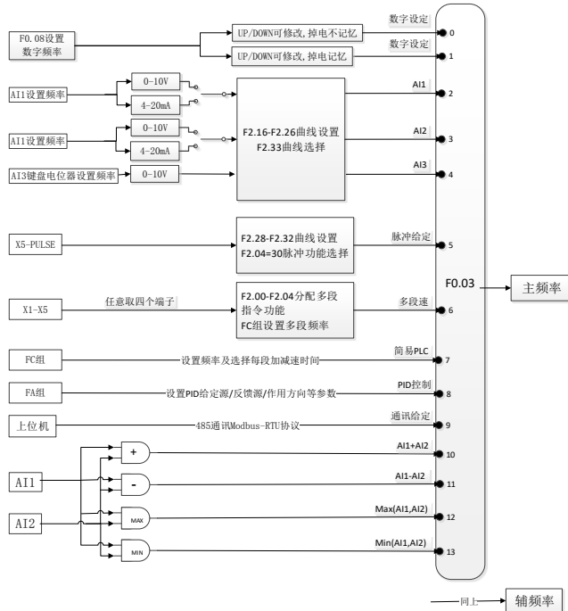
图 5-5 频率给定方式选择
