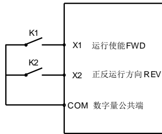
图 7-4 两线运行模式 2
