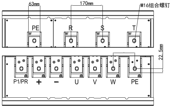
图 3-15 三相 355-450kW 主回路端子分布及尺寸图
