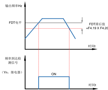
图 7-10 频率 FDT 示意图
