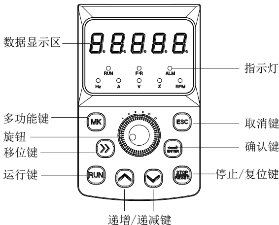
图 4-1 键盘示意图
