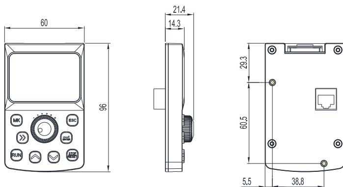
图 1-9 键盘外观及安装尺寸 (mm)
