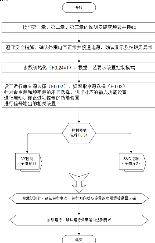
图 5-1 快速调试步骤指南
