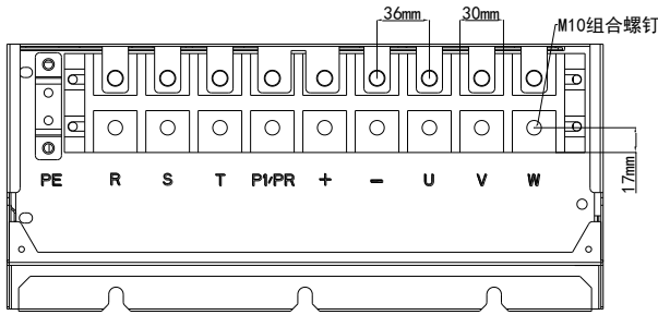
图 3-11 三相 75-90kW 主回路端子分布及尺寸图
