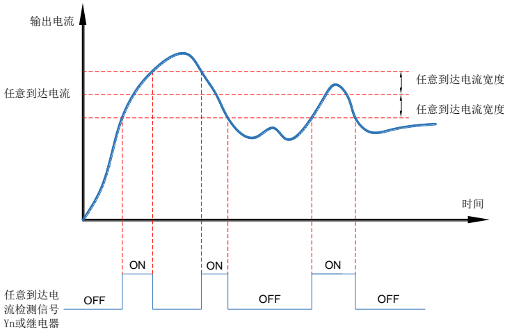
图 7-16 任意电流到达示意图
