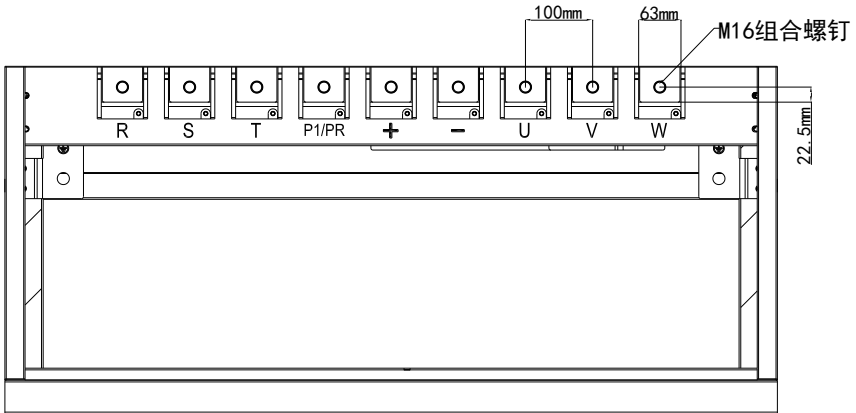
图 3-16 三相 500-560kW 主回路端子分布及尺寸图
