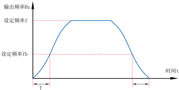
图 7-21 S 加减速曲线 B 示意图
