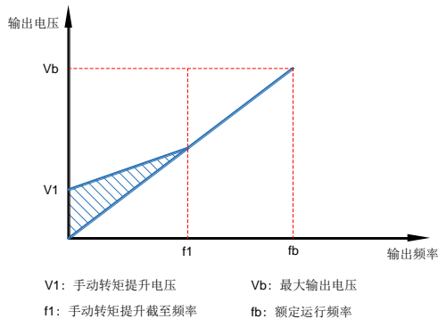
图 7-18 转矩提升示意图
