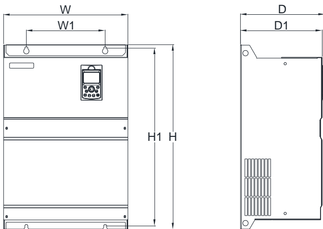
图 1-6 钣金机器安装尺寸
