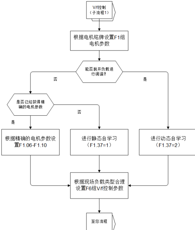
图 5-2 变频器调试子流程 (V/f 控制)
