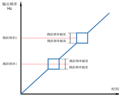
图 7-8 跳跃频率示意图
