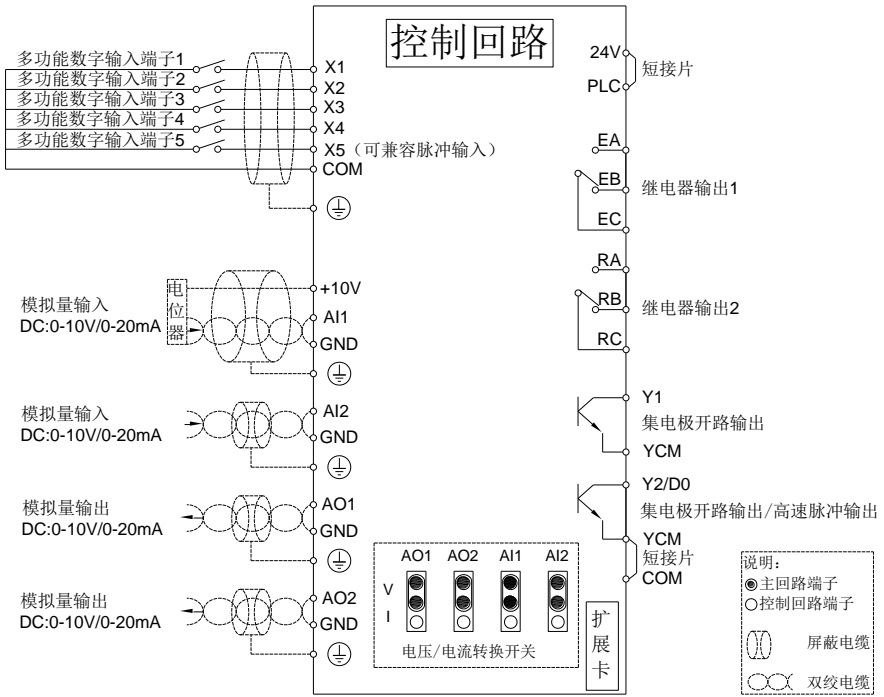
图 3-3 变频器控制回路典型接线示意图
