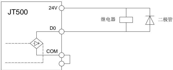
图 3-23 数字输出端子接线示意图
