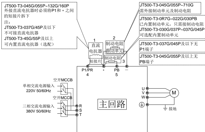
图 3-2 变频器主回路典型接线示意图
