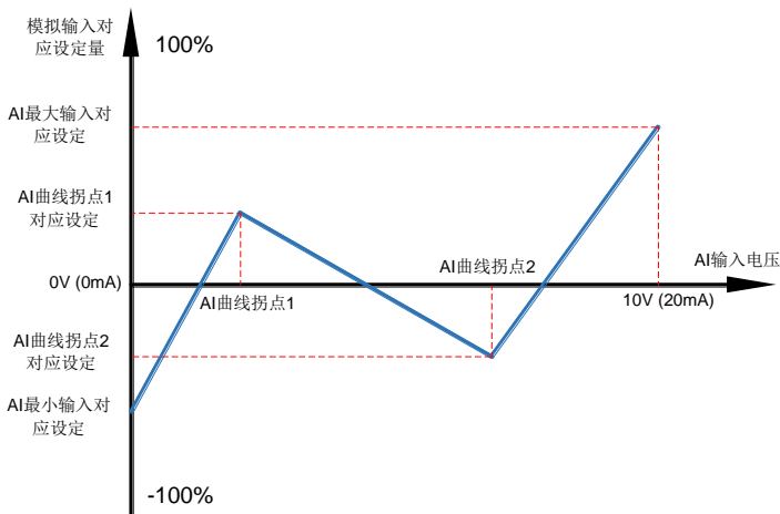
图 6-29 模拟量输入四点偏置示意图
