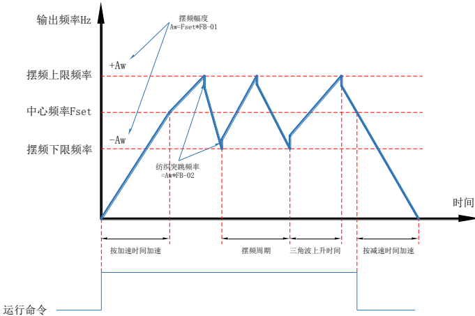
图 7-26 摆频功能示意图
