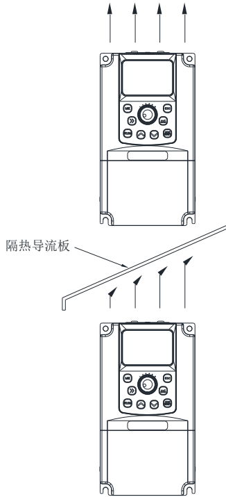
图 2-1 JT500 变频器安装示意图
