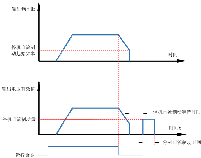
图 7-22 停机直流制动示意图
