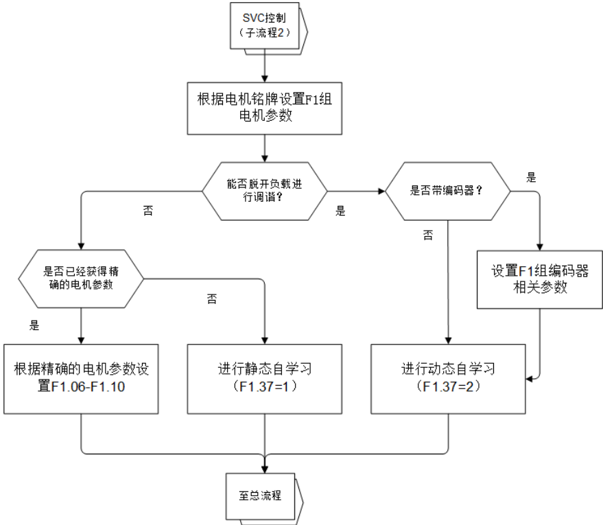
图 5-3 变频器调试试子流程（矢量控制）
