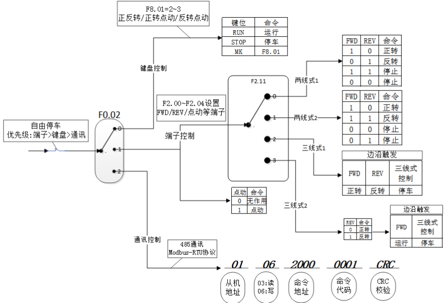
图 5-4 运行命令给定方式选择
