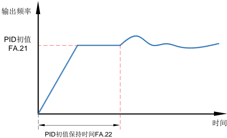
图 7-25 PID 初值保持示意图
