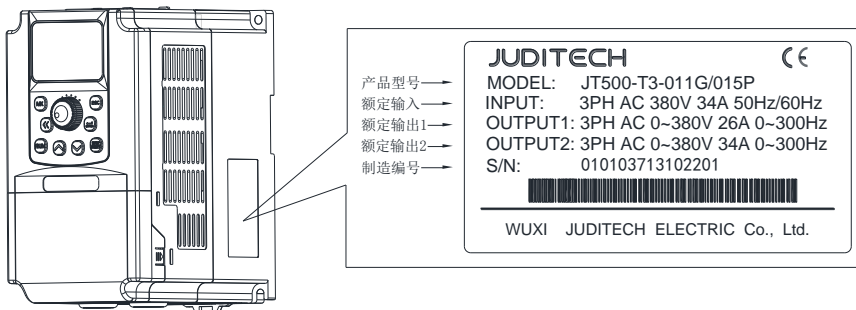
图 1-2 产品铭牌
