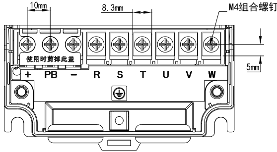
图 3-5 三相 0.75-2.2kW 主回路端子分布及尺寸图
