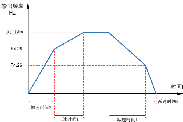
图 7-12 加减速时间切换示意图
