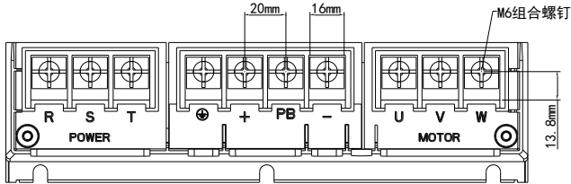
图 3-9 三相 30-37kW 主回路端子分布及尺寸图
