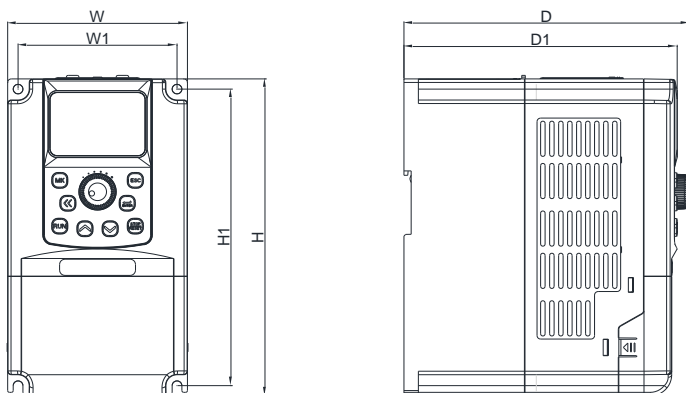
图 1-5 塑壳机器安装尺寸
