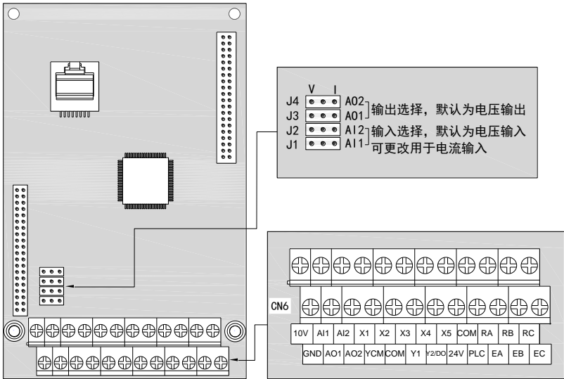
图 3-18 控制回路端子布置图
