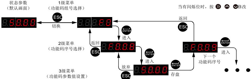
图 4-3 三级菜单操作流程
