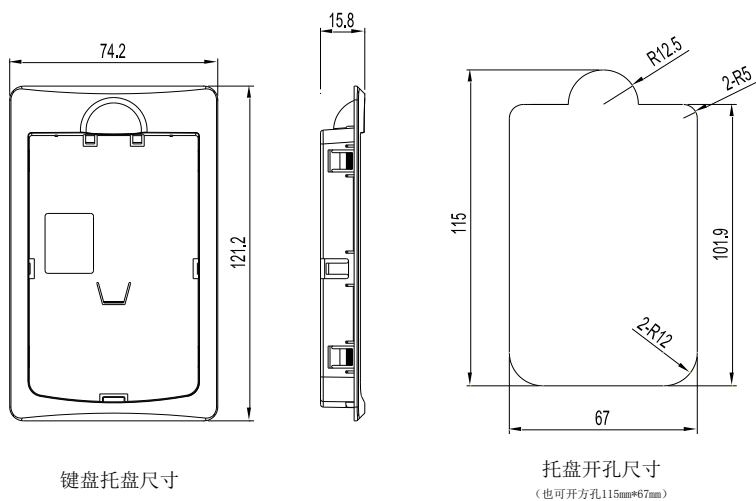
图 1-10 键盘托盘外观及开孔尺寸 (mm)
