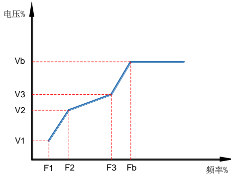
V1-V3: 多段速V/F第1-3段电压百分比 Vb: 电机额定电压 F1-F3: 多段速V/F第1-3段频率百分比 Fb: 电机额定运行频率
