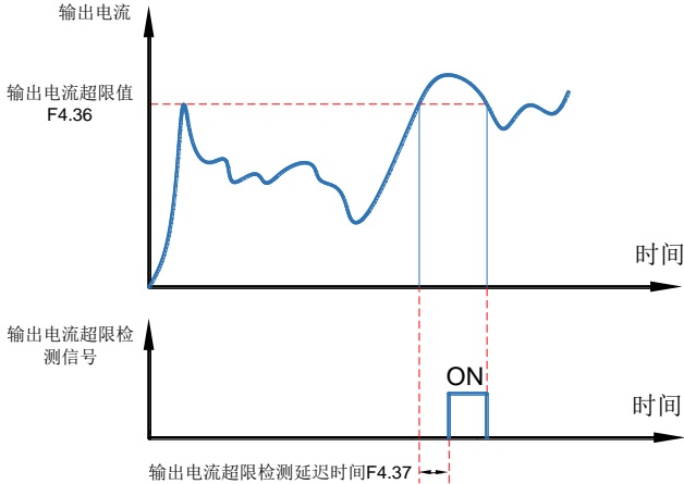
图 7-15 输出电流超限示意图
