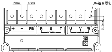
图 3-8 三相 15-22kW 主回路端子分布图
