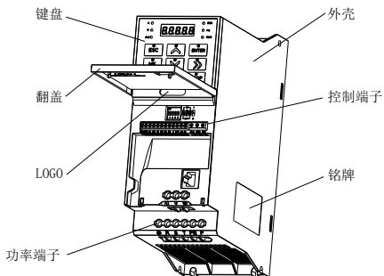
图 1-3 外壳机型各部分名称
