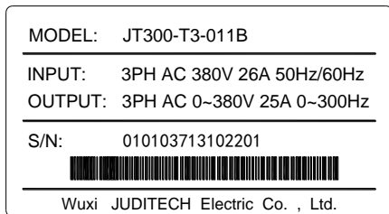
图 1-2 产品铭牌
