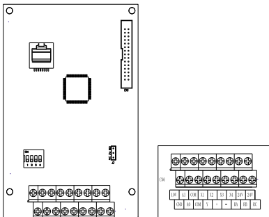
图 3-16 55-132kW 控制回路端子分布图
