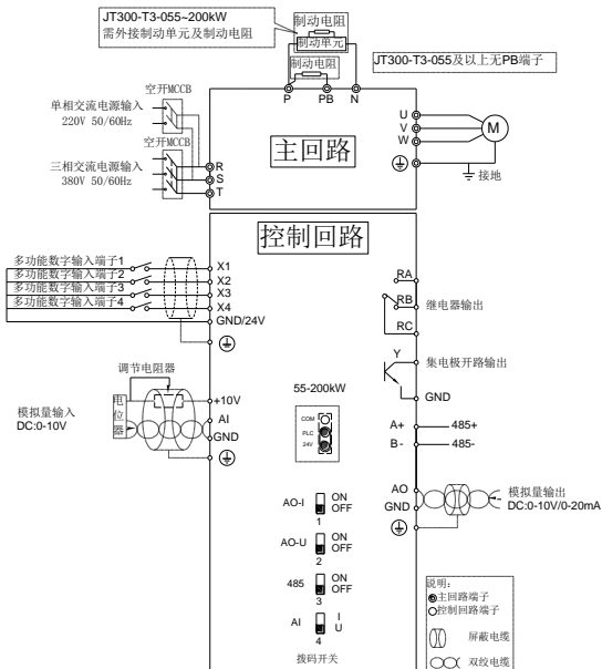
图 3-3 变频器 55-132kW 接线示意图
