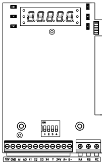
图 3-14 0.75-11kW 控制回路端子分布图
