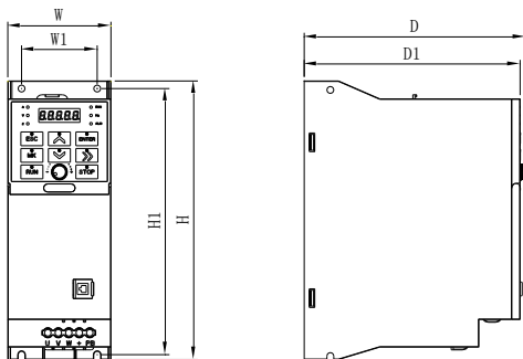
图 1-4 塑壳安装尺寸
