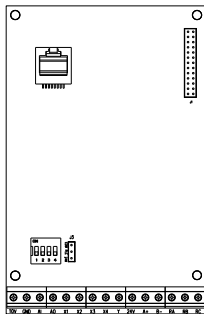
图 3-15 15-45kW 控制回路端子分布图
