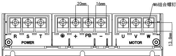
图 3-9 三相 30-37kW 主回路端子分布图
