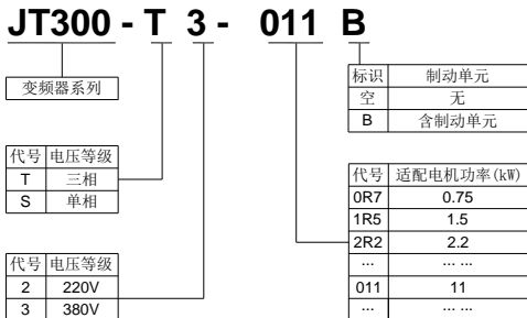
图 1-1 产品命名
