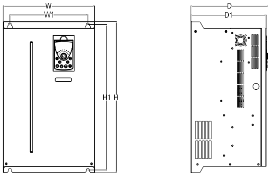
图 1-5 钣金安装尺寸
