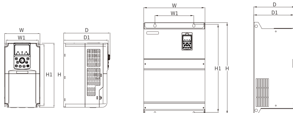
塑壳变频器安装尺寸图
