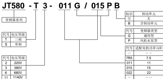
图 1-1 产品命名
