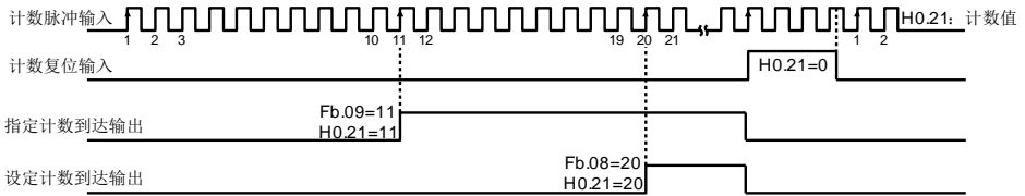
图 6-27 计数功能示意图
