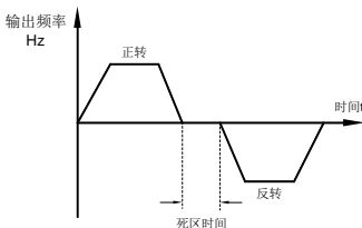
图 6-9 正反转死区时间示意图
