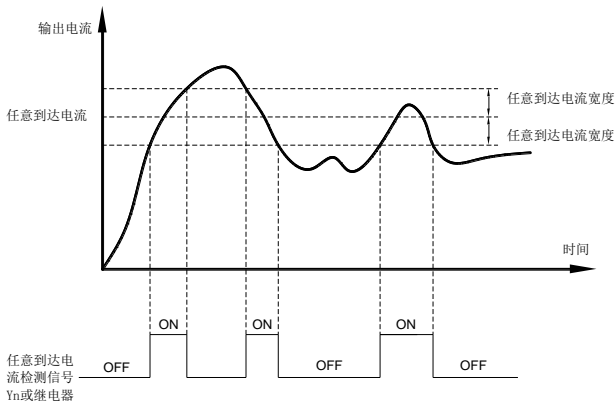
图 6-16 任意电流到达示意图
