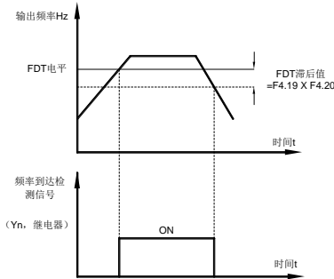
图 6-10 频率 FDT 示意图
