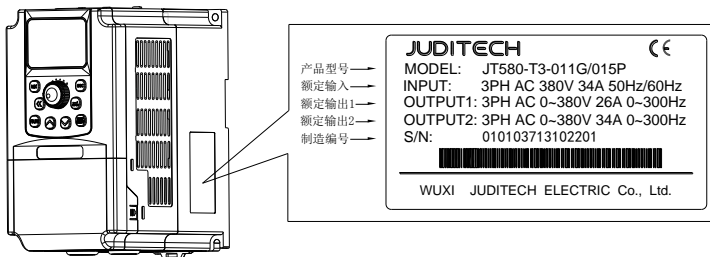
图 1-2 产品铭牌
